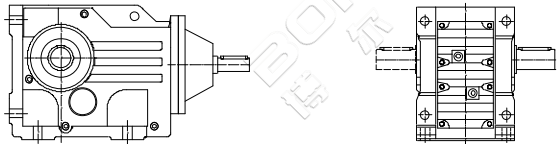
K (KF, KA, KAF, KAB, KAZ) S... 轴输入的螺旋锥齿轮减速机 Shaft input helical-bevel gear units
