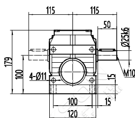
S47
