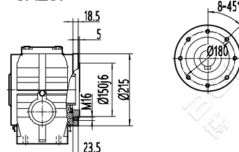
SAZ87
