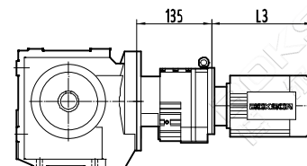
S..37R17
