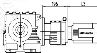
S..87R57
