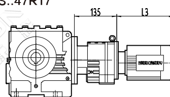
S..47R17
