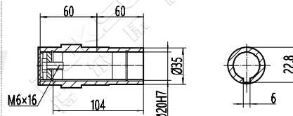
S..37R17
