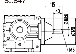
S..S47
