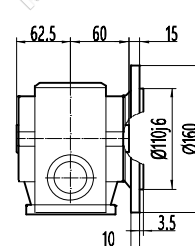
SAF37/Φ160
