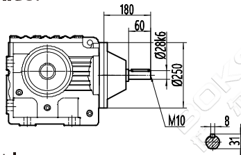
S..S87
