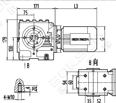
SA47
