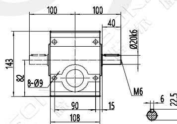
S..S37
