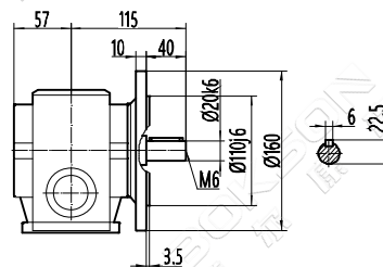
SF37/Φ160
