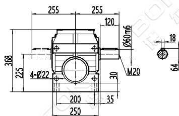
S87
