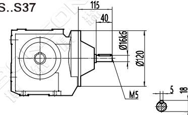
S..S37
