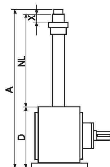
输入锥齿轮装配型式 (5种)
