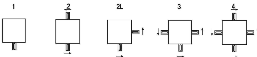
输入锥齿轮装配型式 (5种)
